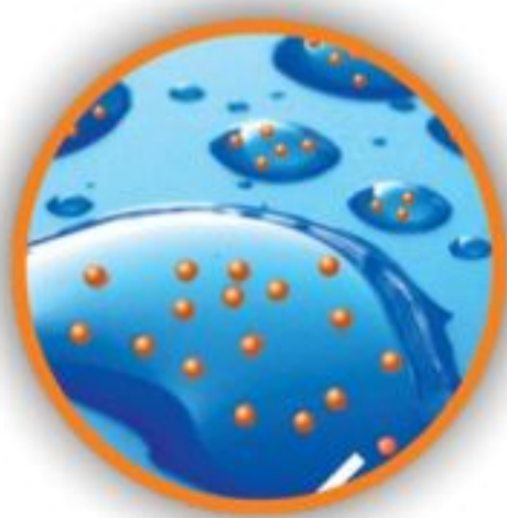
Macromoléculas
